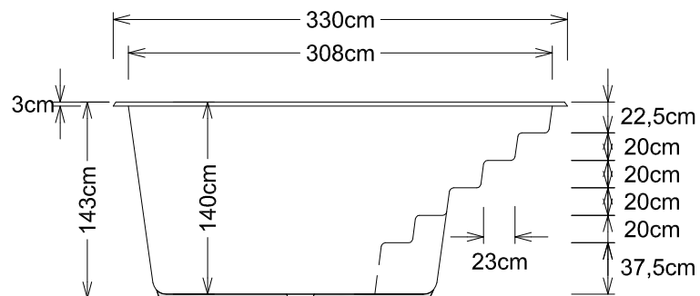
Schnitt - Sezione B - B
