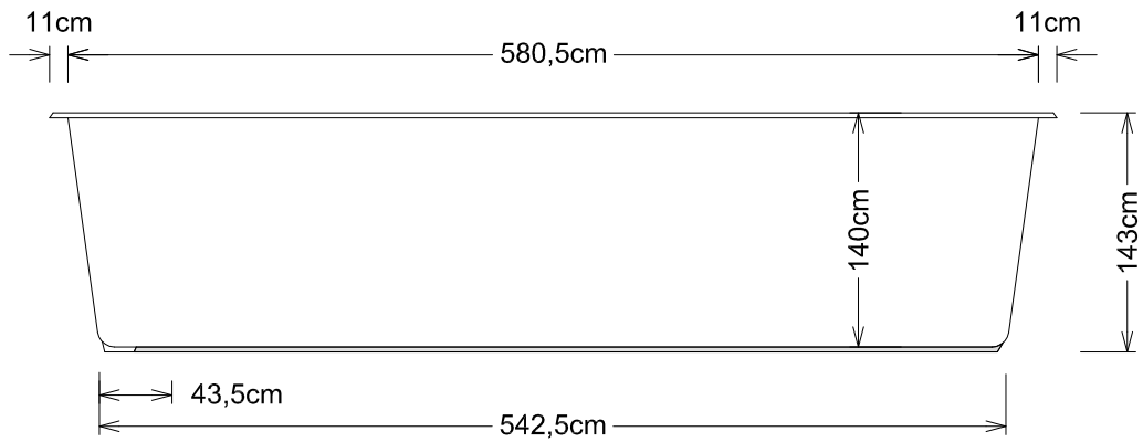
Schnitt - Sezione A - A
