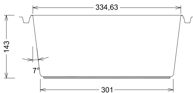
Querschnitt
