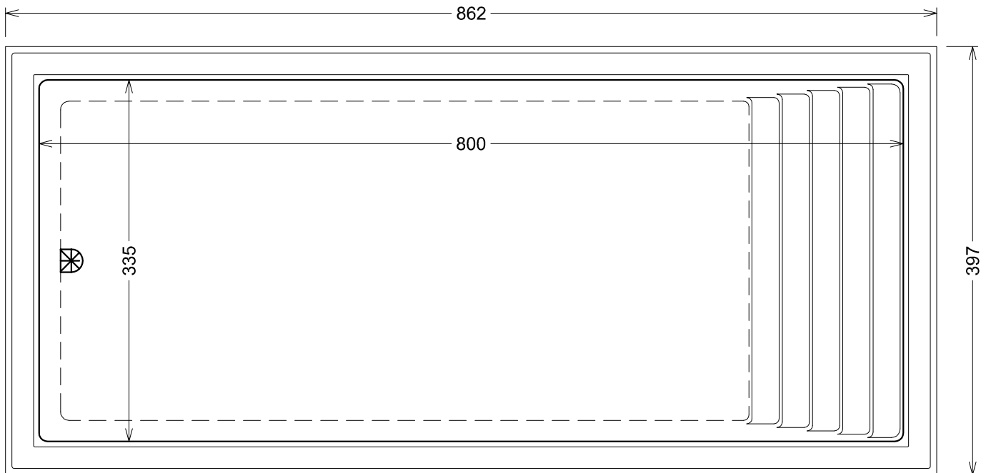
Grundriss
