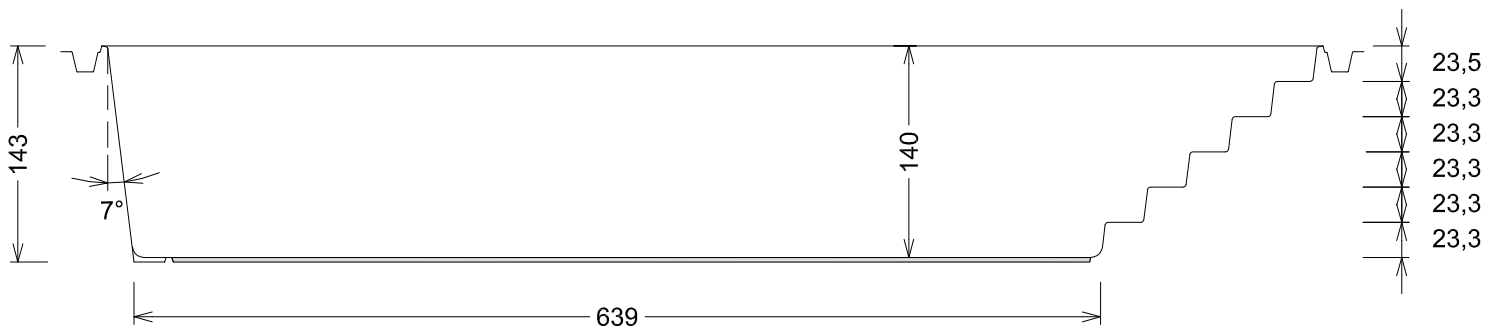
Längsschnitt
