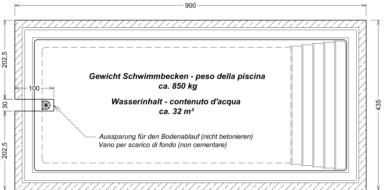
Grundriss
